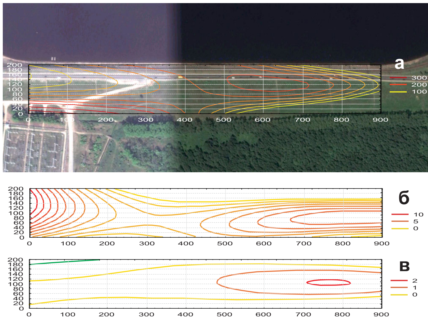
Рис. 4. Изменения содержания ионов в аллювиальном водоносном горизонте, мг/л: а — \text{HCO}_3^- ; б — \text{NH}_4^+ ; в — \text{Fe}^{2+} . Вертикальные оси — расстояние, м; горизонтальные оси — расстояние, м; изолинии разных цветов соответствуют разной концентрации указанных ионов, мг/л (см. легенды справа от рисунков)
