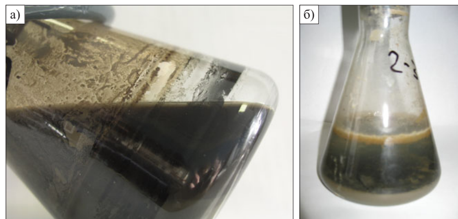
Рис. 3. Образование осадков черного и охристого цвета в результате развития в грунте микроорганизмов: а — осадок черного цвета на стенках колбы вблизи дна; б — осадок охристого цвета на стенках колбы вблизи границы раздела «среда — воздух»
