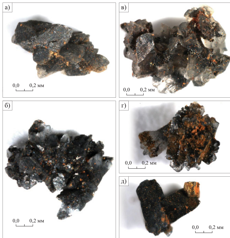
Рис. 2. Техногенные минералы донных отложений колодца вертикального дренажа: а — зерна кальцита с идиоморфными гранями и ступенчатой поверхностью спайности; б — затемненный в центре и прозрачный по краям агрегат кристаллов кальцита; в — агрегат прозрачных зерен кальцита; г — агрегат кристаллов кальцита с налетом гидроксидов железа (III) на поверхности; д — срастание зерен кальцита и пирита
