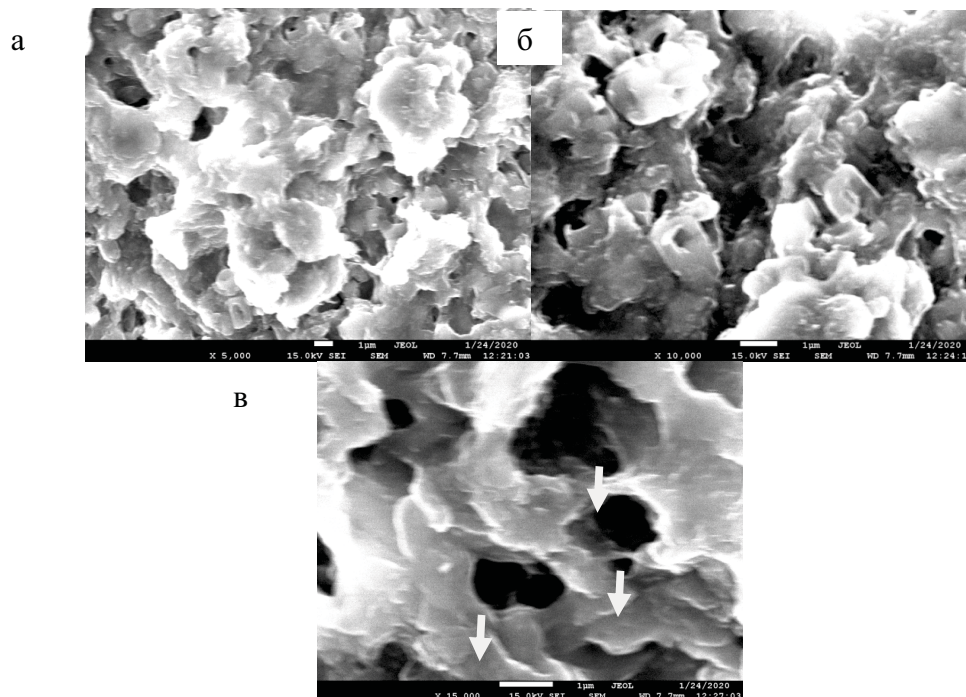
Рис. 3. Электронно-микроскопическое изображение поверхности образца 3: а) увеличение \times 5000 , б) увеличение \times 10000 , в) увеличение \times 15000 ; стрелками отмечено формирование связей между микроагрегатами
