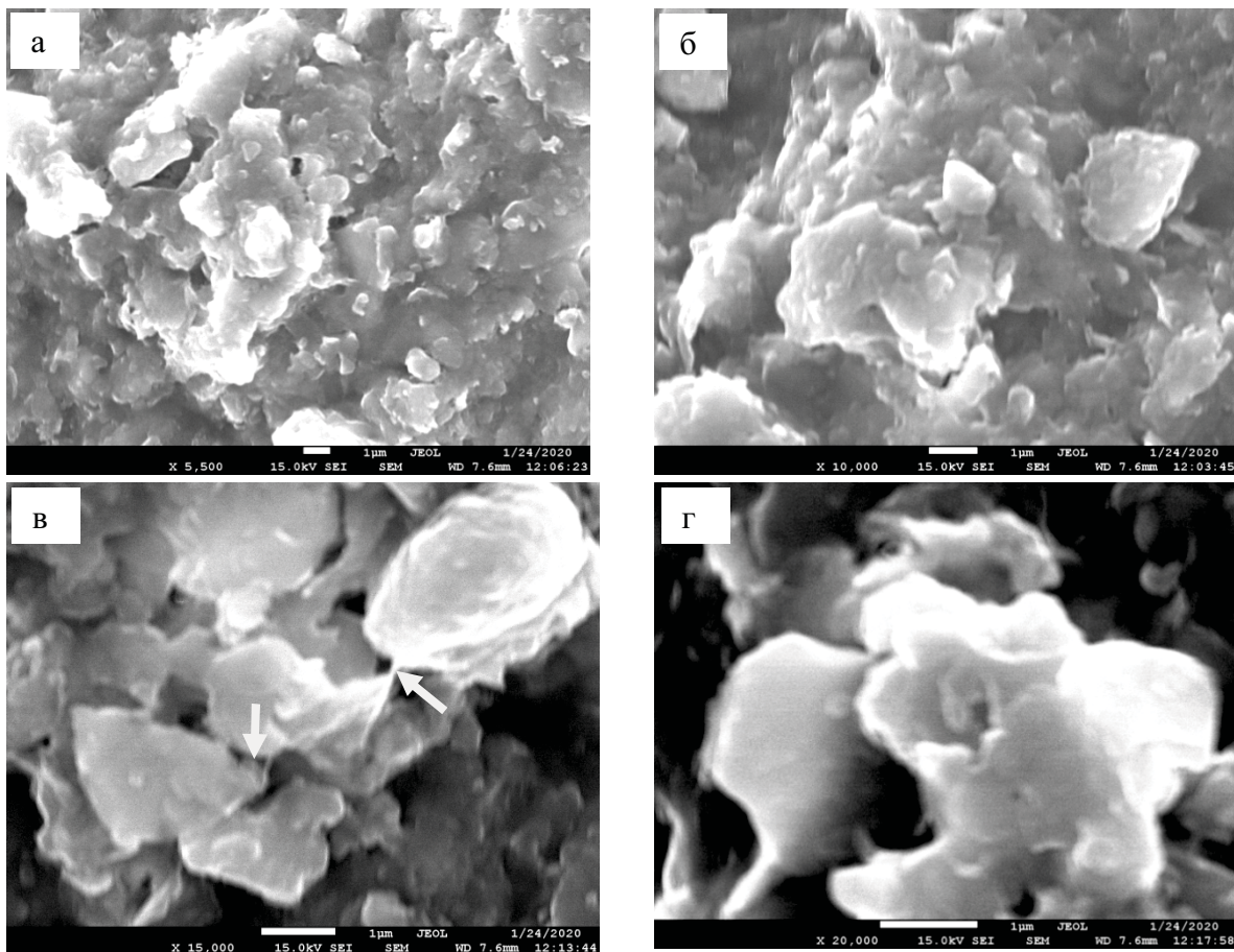
Рис. 2. Электронно-микроскопическое изображение поверхности образца 2: а) увеличение \times 5000 , б) увеличение \times 10000 , в) увеличение \times 15000 , г) увеличение \times 20000 ; стрелками отмечено формирование связей между микроагрегатами)
