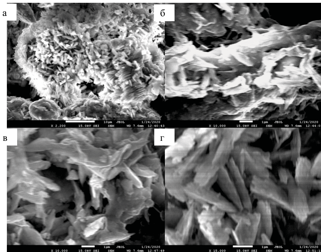
Рис. 4. Электронно-микроскопическое изображение поверхности образца 4: а) увеличение \times 2200 , б) увеличение \times 10000 , в) увеличение \times 10000 , г) увеличение \times 15000 ;
