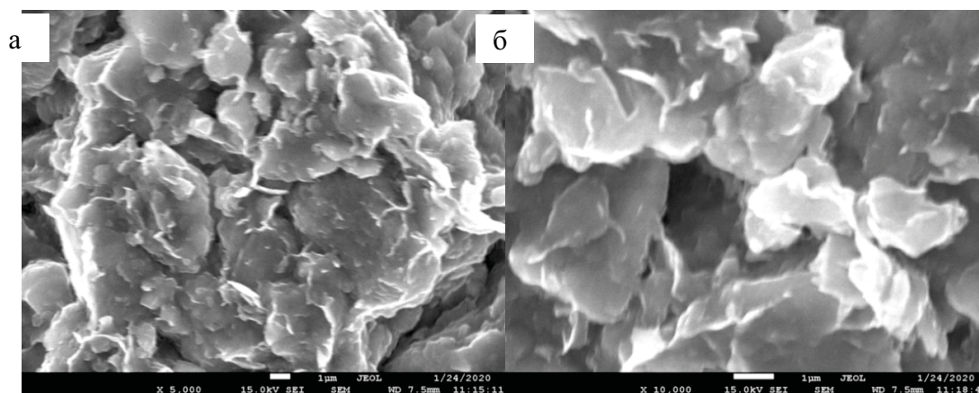
Рис. 1. Электронно-микроскопическое изображение поверхности образца 1: а) увеличение \times 5000 , б) увеличение \times 10000
